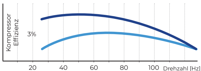
Stufenlose Drehzahlregelung zwischen 1200 - 7200 l/min
